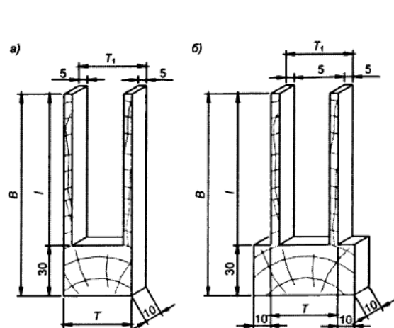
Рис. 6. Силовой образец для пиломатериалов толщиной а — до 40 мм и б — более 40 мм. В — ширина доски
